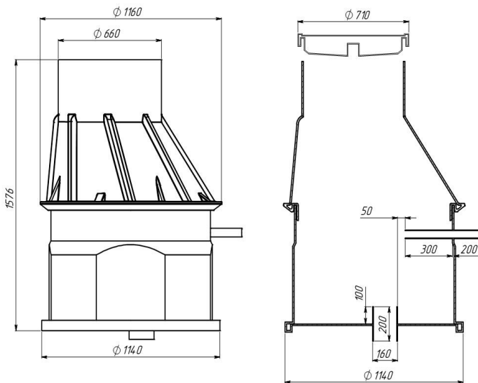
Кесон плоскодонный
