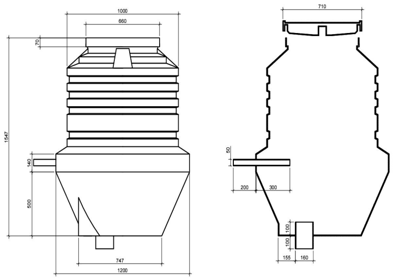
Кесон конический
