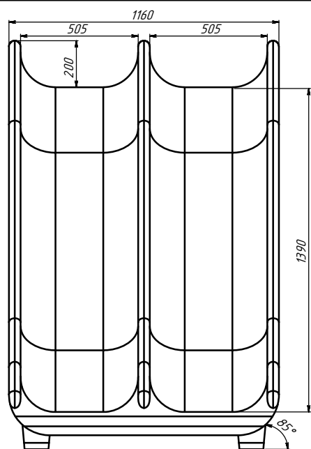
Вид А МАСШТАБ 1 : 10 повернуто
