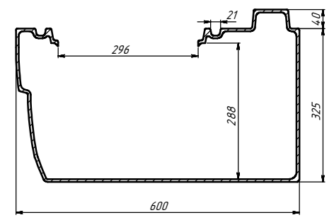
СЕЧЕНИЕ А-А МАСШТАБ 1 : 4
