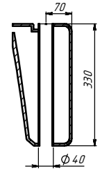
СЕЧЕНИЕ А-А МАСШТАБ 1 : 5
